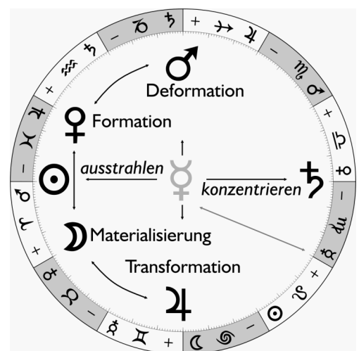
die Erhöhungen
