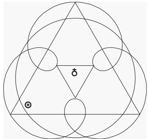
geozentrische Merkurbahn
