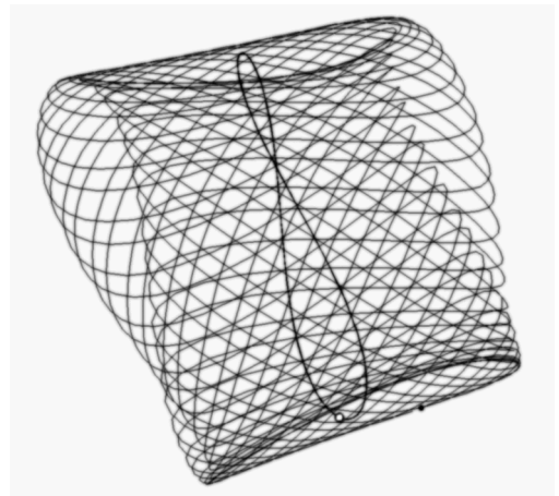
Organform Merkur-Sonne 2000-2012
